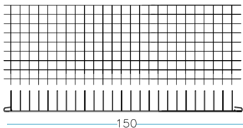
nr. 2 pz. Laterale lungo 150 x H. 50 cm
